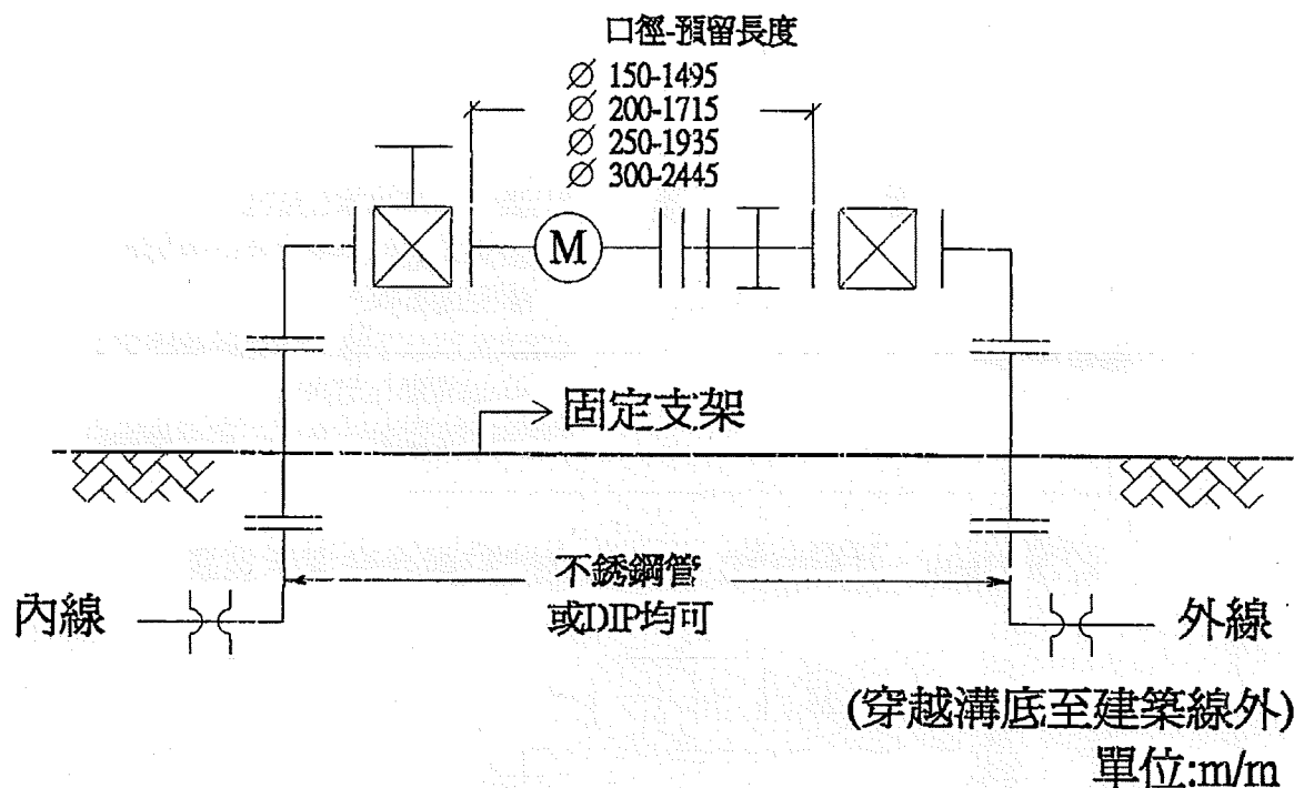
φ 150m/m(含)以上水量計地上式水表組按裝組合參考尺寸示意圖
